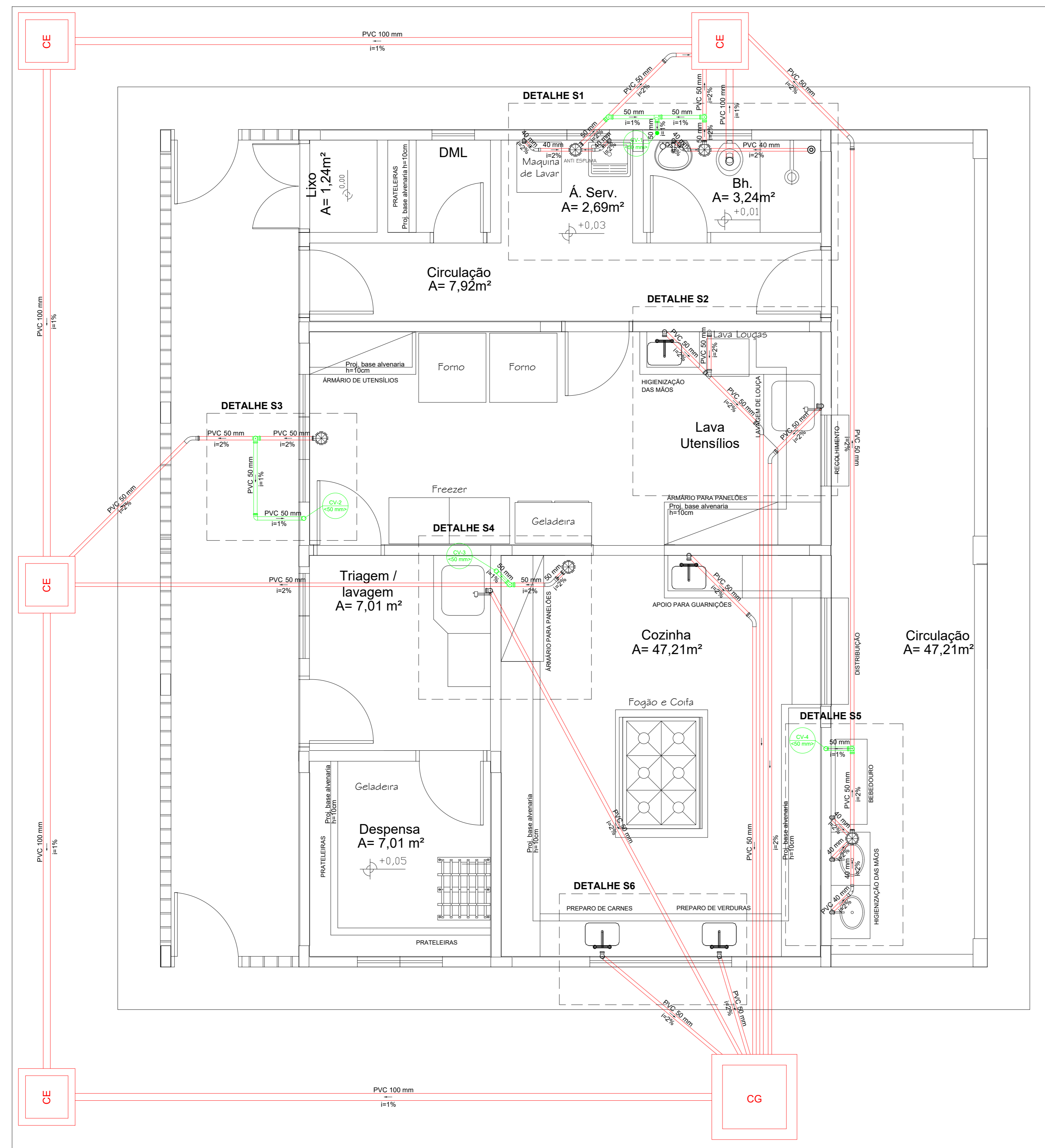
Planta do Terreo - Esgoto Escala 1:50
