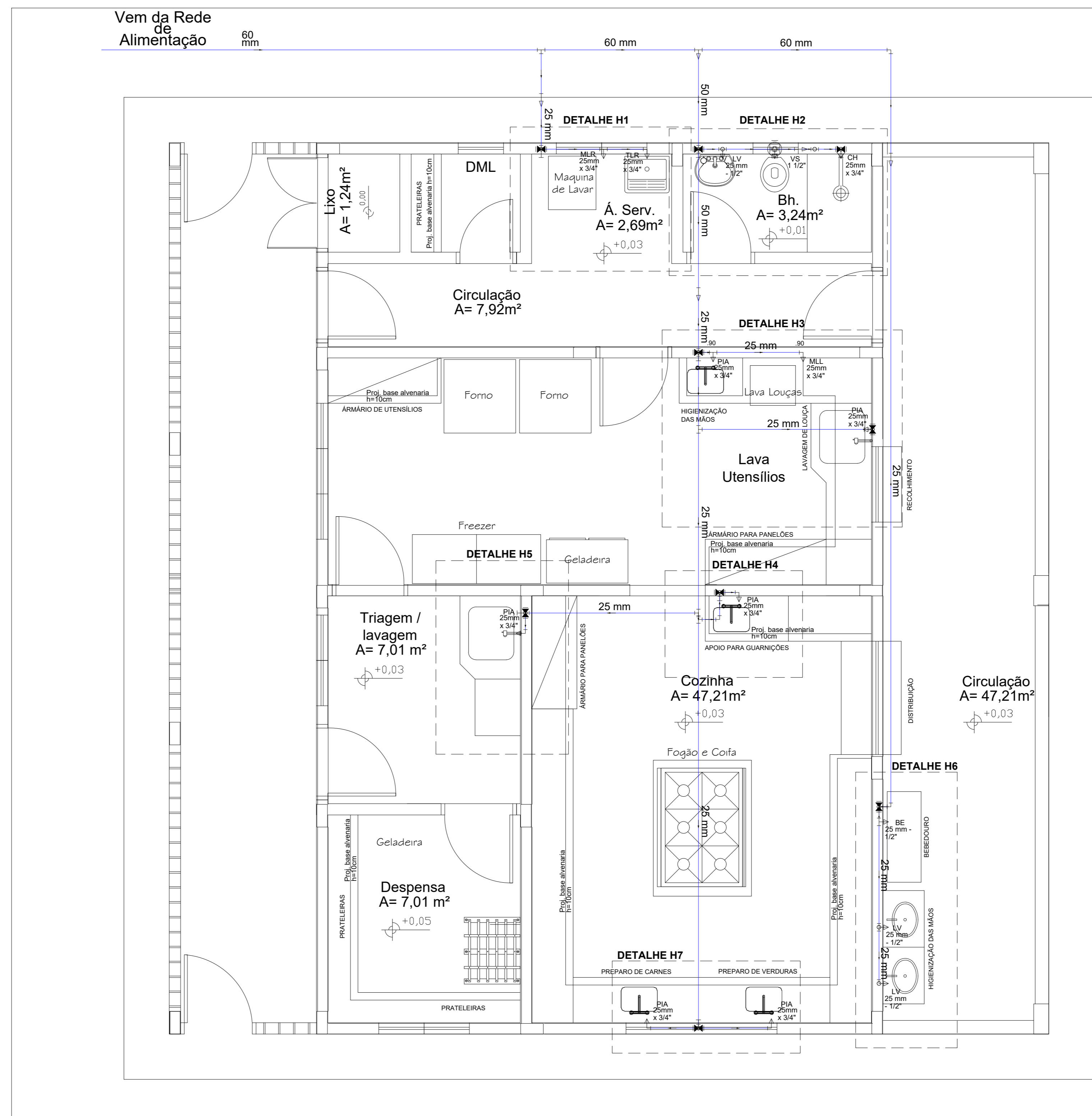
Planta do Terreo - Agua Fria Escala 1:50
